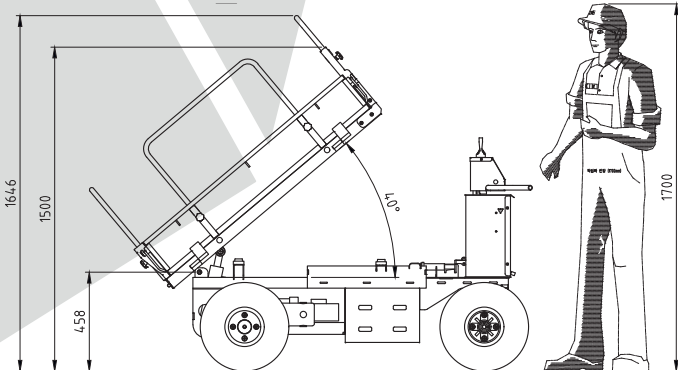
KIT ERHÖHUNG LADEBRÜCKE ART. NR. 3121737 PREIS 144.-
